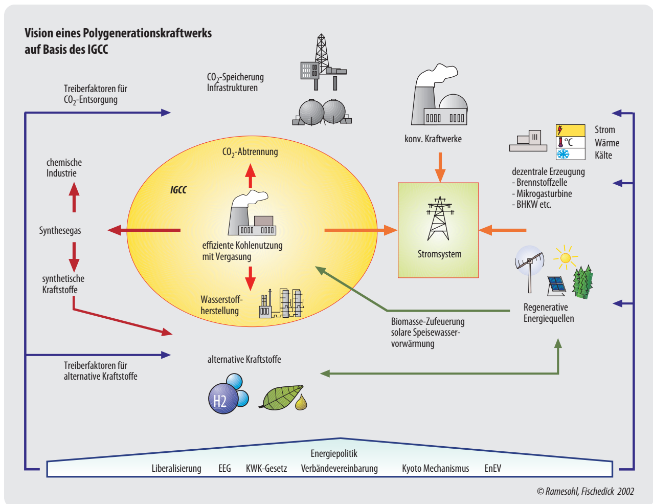
Abbildung 7: Vision eines Polygenerationskraftwerks mit verschiedenen Eingangsprodukten und verschiedenen Ausgangsprodukten auf der Basis der integrierten Vergasungstechnologie (IGCC)
