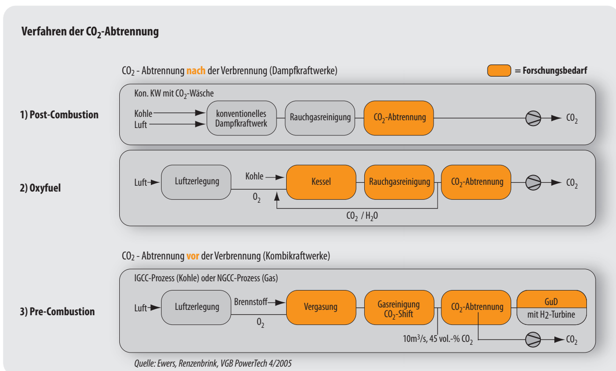
Abbildung 6: CO 2 -Abscheideverfahren im Überblick
