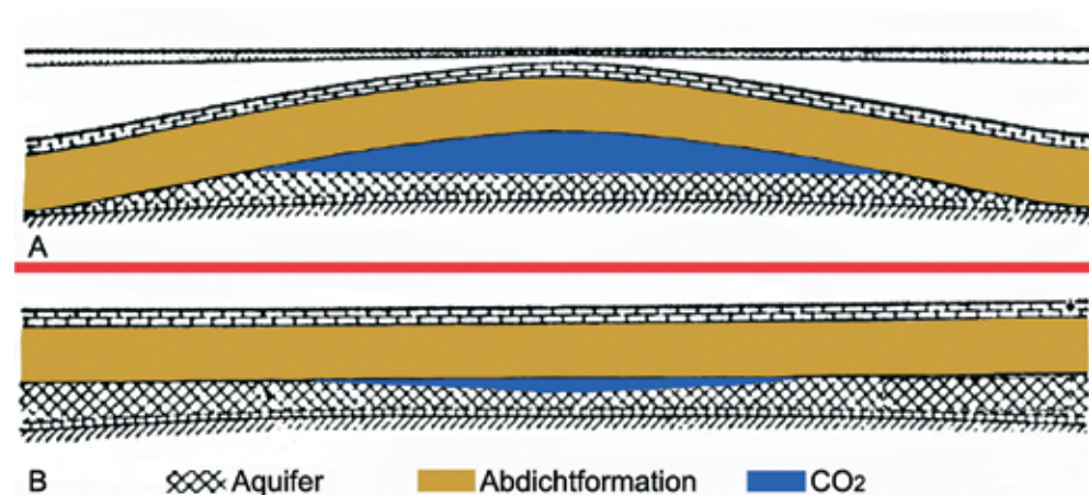
Abbildung 12: Geologische Voraussetzungen für eine stabile Speicherung Fall A: Stratigraphische und Strukturelle Falle, Fall B: Stratigraphische Falle (WI/GD 2006)
